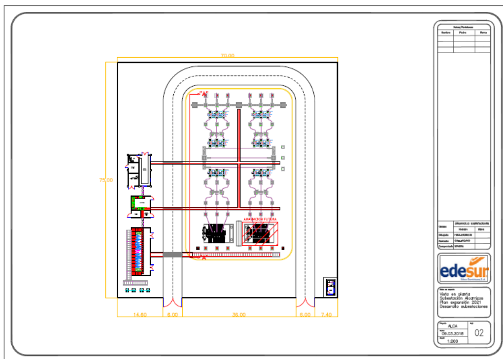
Figura 2. Vista en planta propuesta S/E Los Alcarrazos.
