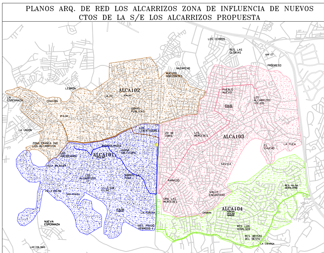
Imagen 2. Área de influencia de circuitos de subestación Piedra Blanca.
