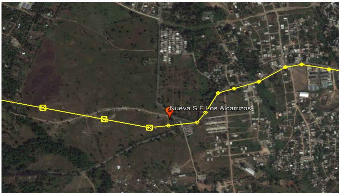
Ubicación propuesta subestación Los Alcarrazos con la línea de transmisión 138 kV existente.
